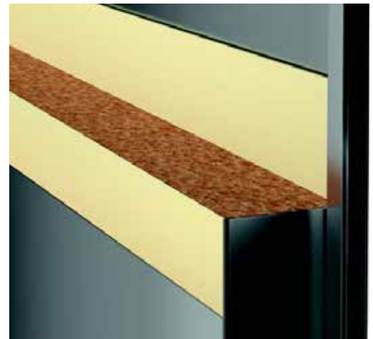
Türblatt in vollflächig verklebter Verbundkonstruktion
