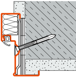
Diagonalbefestigung (Mauerwerk)
